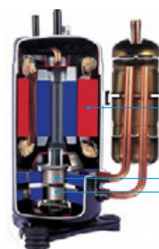
Компрессор (двухроторный)
