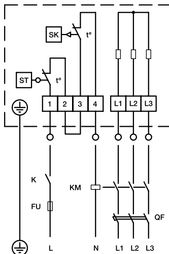
Схема подключения 4 Круглый канальный нагреватель на 400 В (3 фазы)
