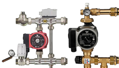
Узлы смешения
