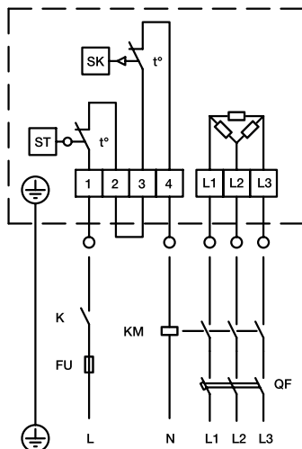
Схема подключения 3 Круглый канальный нагреватель на 400 В (3 фазы)
