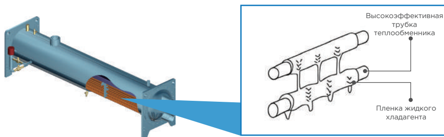
Схема испарителя со сплошной нисходящей пленкой
