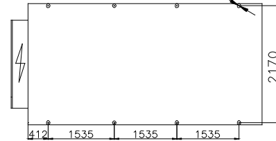
Схема расположения виброопор. 8 отверстий D14 для крепления виброопор
