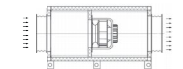
6. Напольные/подвесные вытяжные установки.
