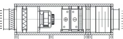
9. Напольные/подвесные приточные установки с водяным нагревателем, водяным охладителем и секцией шумоглушителя.
