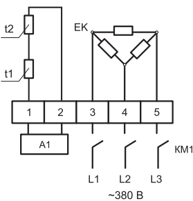
Схема подключения STE-3 Круглый канальный нагреватель на 380 В
